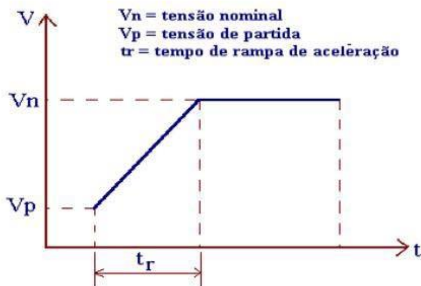
Figura 4 – Curva de aceleração de um MIT usando soft-starter
