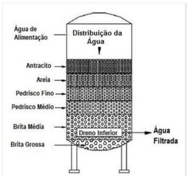
Filtração Multimídia
