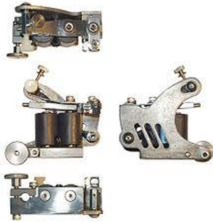
Aparelho elétrico de tatuar.
