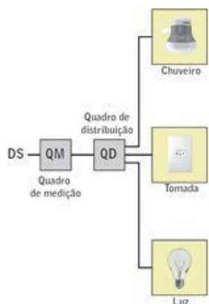
Figura 1 - Casa térrea
